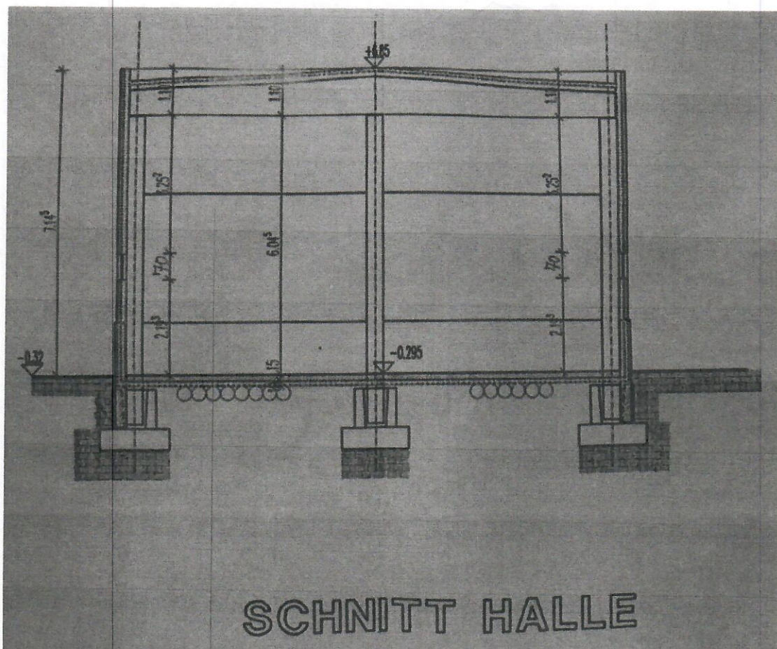
Schnitt Halle – Objekt Ost
