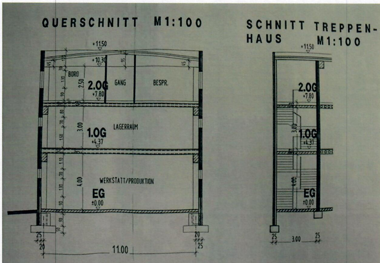
Schnitt – Objekt West
