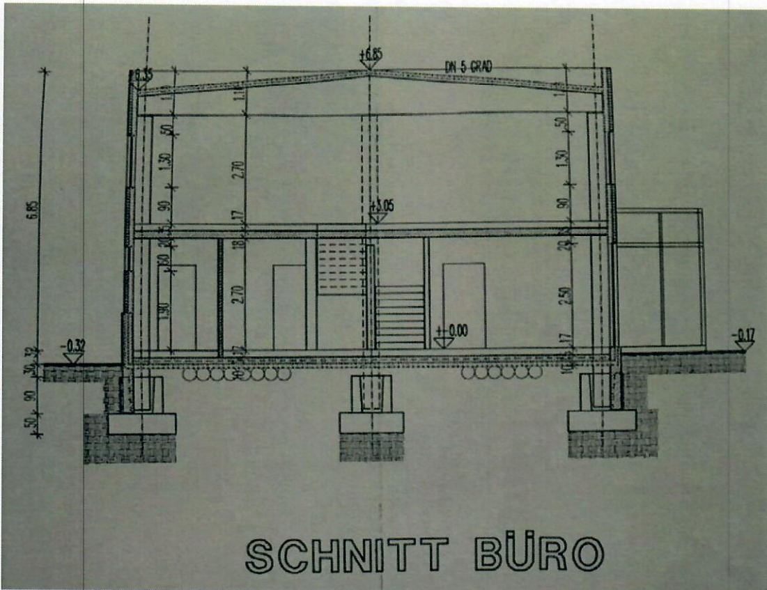
Schnitt Büro – Objekt Ost
