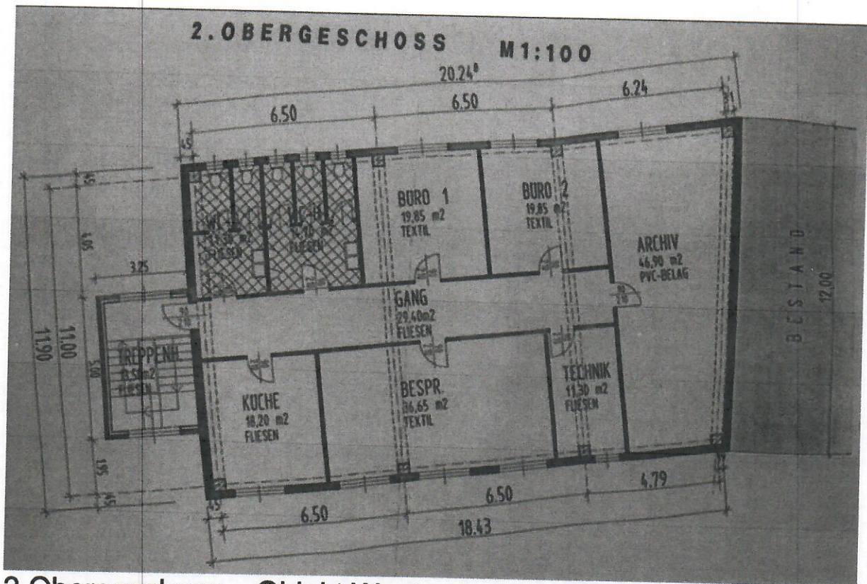
2. Obergeschoss – Objekt West
