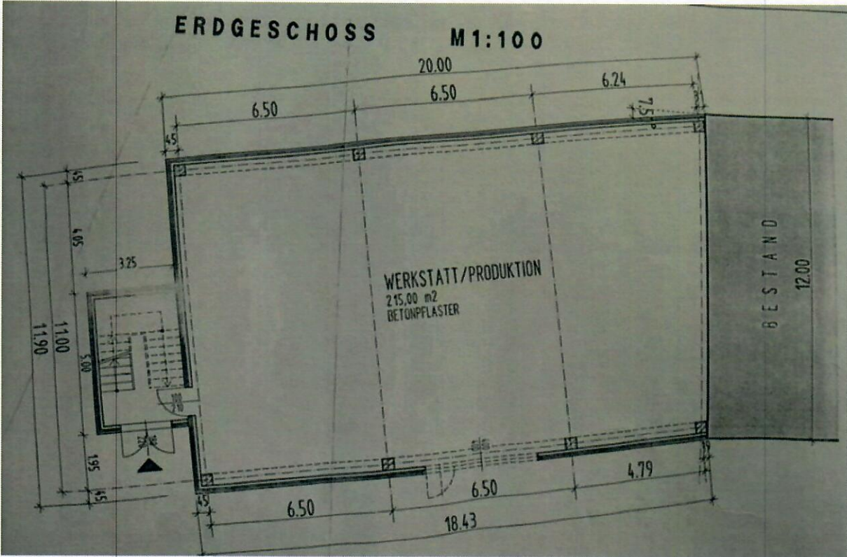
Erdgeschoss – Objekt West
